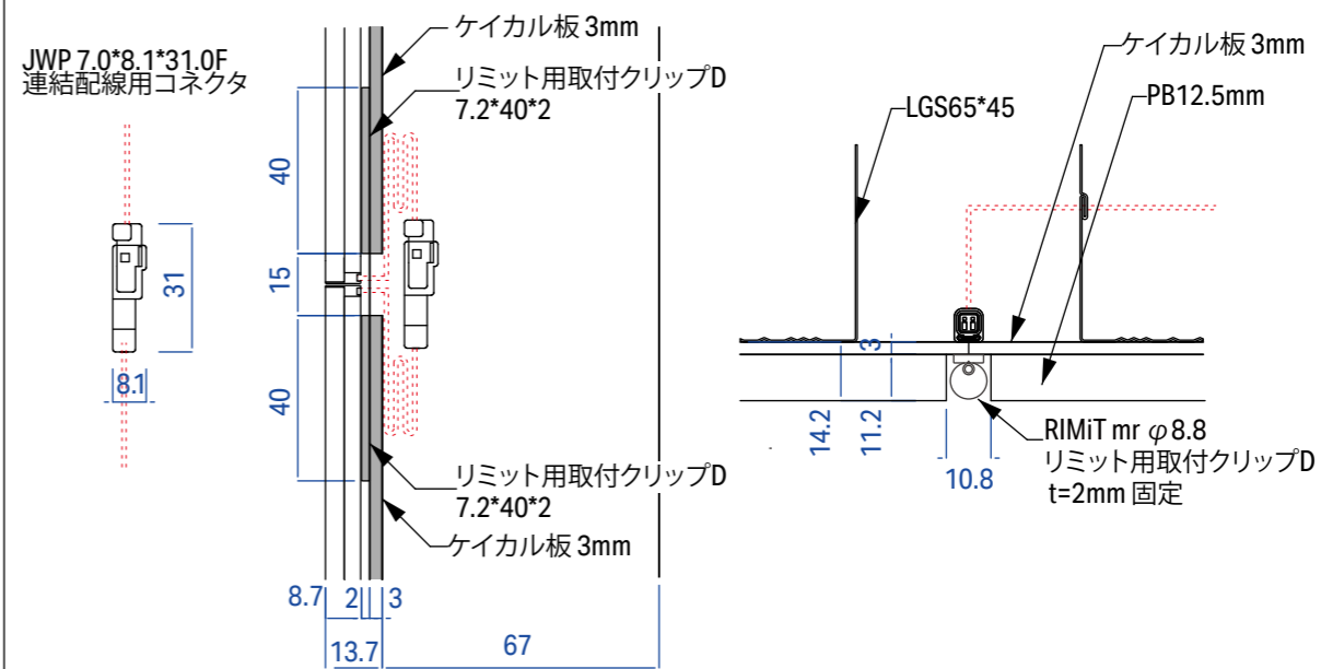
コネクタ連結字詳細図 S=1:2
