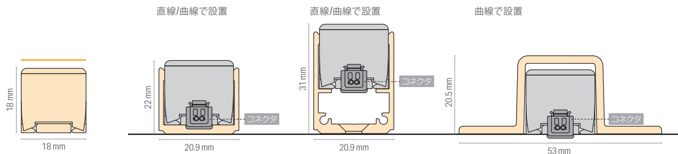
灯具断面サイズ
