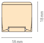
断面サイズ W18 x H18 mm
