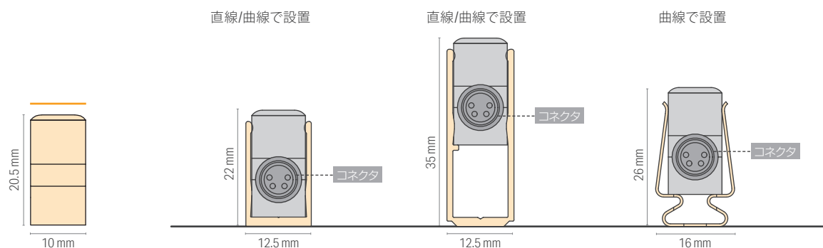
灯具断面サイズ
