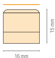
断面サイズ トップビュータイプ (TV) W16 x H15 mm
