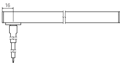
上面図
