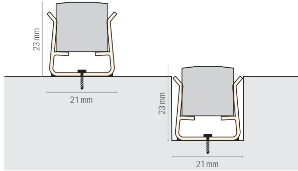
オプション品使用時の断面サイズ
