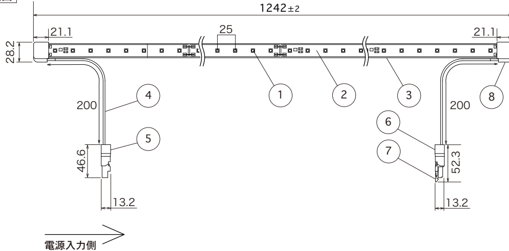
正面図
