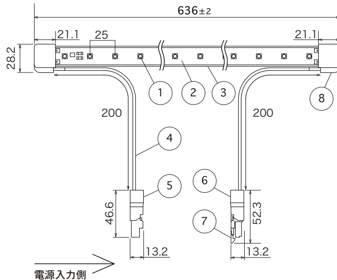
正面図
