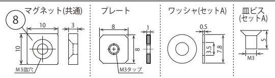
オプション品：マグネットセットR (型番：MG-R：4セット/1箱)
