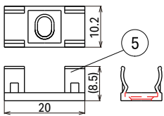
オプション品：リミットmr用取付クリップ (型番：LRMMR-PT-G)(5個/1袋)
