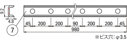
オプション品： リミットフレックスmr用取付レール1000 (型番：LRFM-RL1000)
