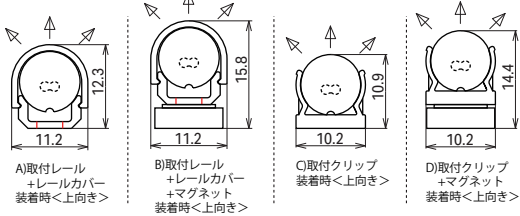
オプション品：リミットmr用取付クリップ (型番：LRMMR-PT-G)(5個/1袋)
