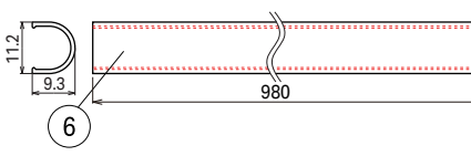
オプション品： リミットフレックスmr用レールカバー1000 (型番：LRFM-C1000)
