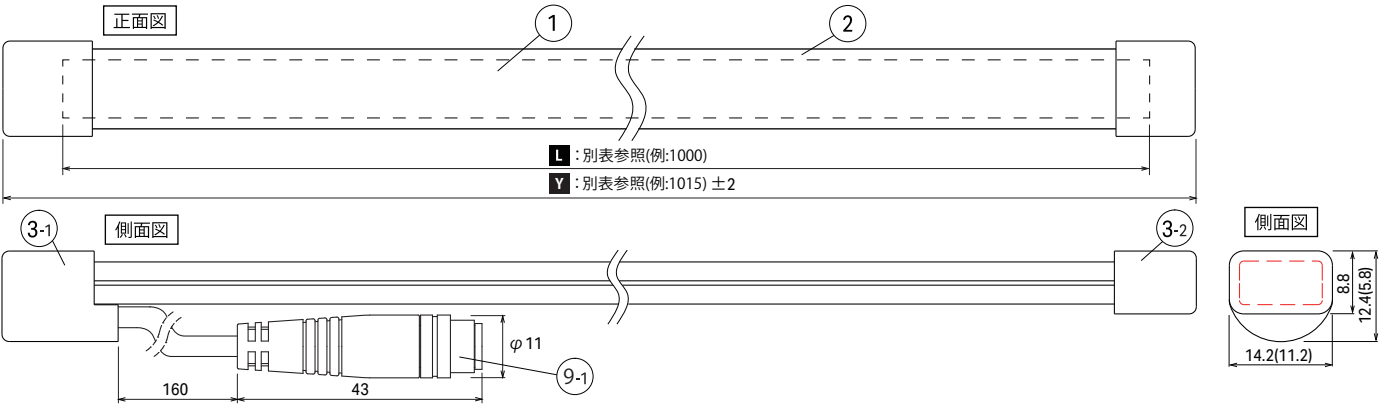
設置寸法 (側面図)
