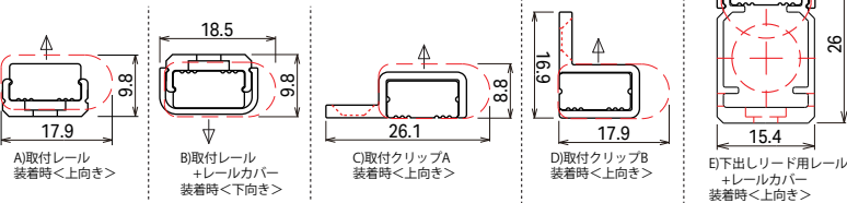
設置寸法 (側面図)
