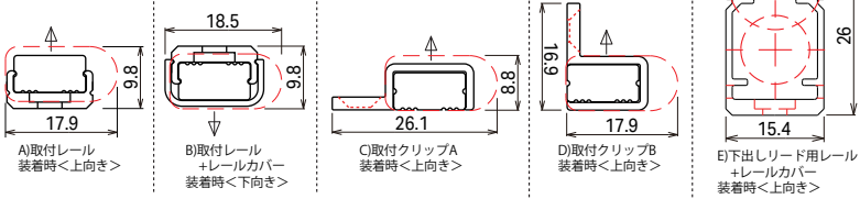
設置寸法 (側面図)
