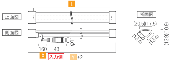
リミット フレックス SOTO sk / 屋外仕様・片側AH1コネクタ・リード線側面出し
