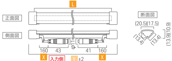
リミット フレックス SOTO sk / 屋外仕様・両側AH1コネクタ・リード線側面出し
