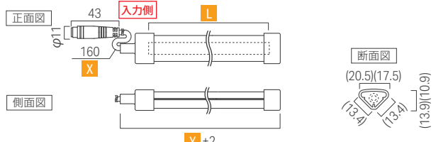
リミット フレックス SOTO sk / 屋外仕様・片側AH1コネクタ・リード線側面出し
