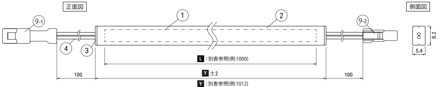
設置寸法（側面図）
