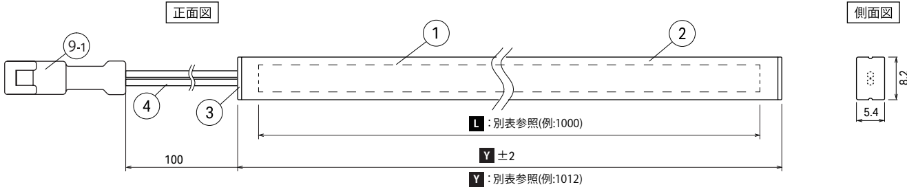
設置寸法 (側面図)
