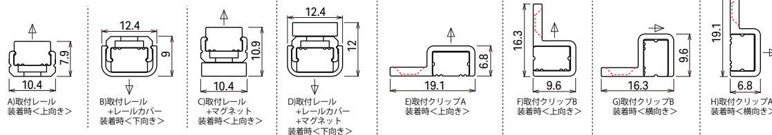
設置寸法（側面図）
