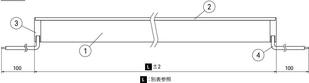
側面図
