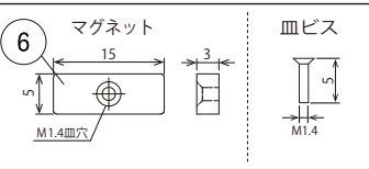
オプション品：マグネットセットH (型番：MG-H：5セット/1箱)
