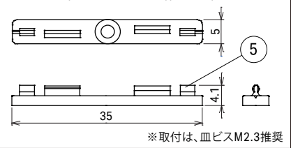
オプション品：リミットhs用取付クリップ (型番：LRMHS-PT-N)(5個/1袋)
