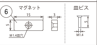
オプション品：マグネットセットH (型番：MG-H：5セット/1箱)
