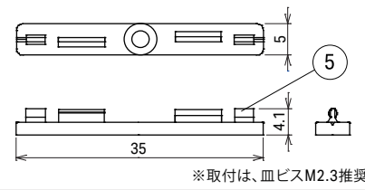
オプション品：リミットhs用取付クリップ (型番：LRMHS-PT-N)(5個/1袋)
