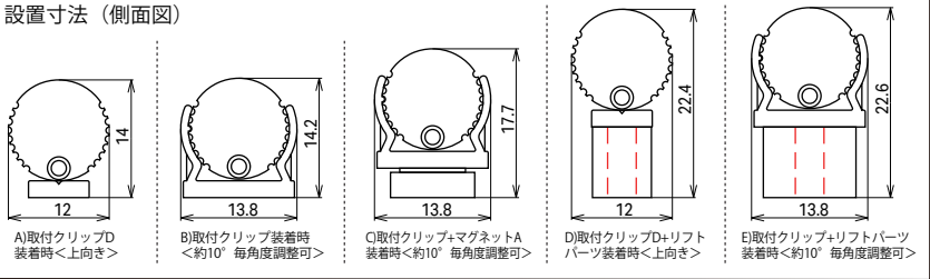
オプション品： リミットlens用取付クリップ (型番：LRMLE-PT-P)(5個/1袋)
