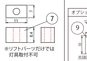
オプション品： リミット用リフトパーツ (型番：LRM-PT-B)(5個/1袋)
