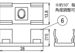
オプション品： リミットlens用取付クリップ (型番：LRMLE-PT-P)(5個/1袋)
