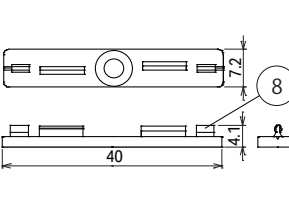
オプション品： リミット用取付クリップD (型番：LRM-PT-D)(5個/1袋)
