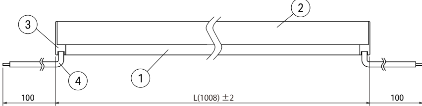
側面図
