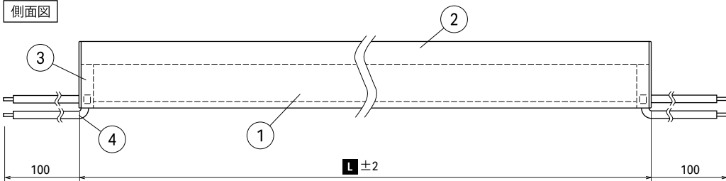
側面図
