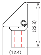
C)取付クリップ +リフトパーツ 装着時<上向き>
