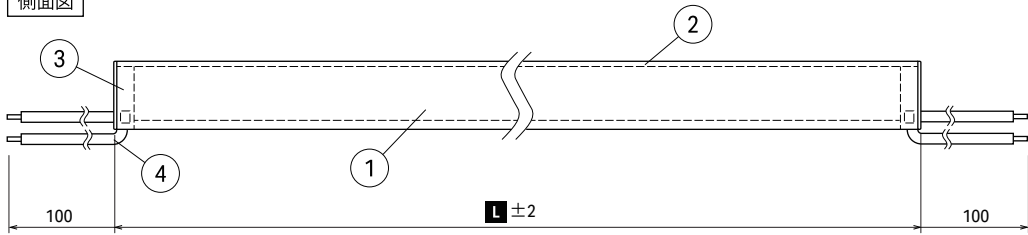
側面図
