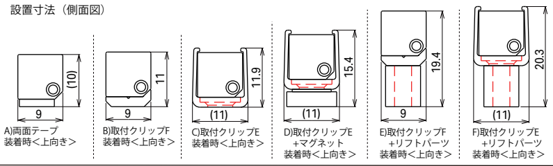
設置寸法 (側面図)
